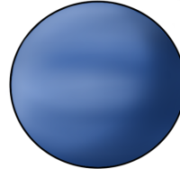
NEPTŪNUS
