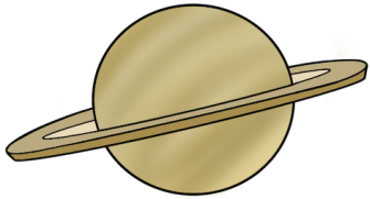
SĀTURNUS
