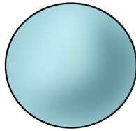
ŪRANUS
