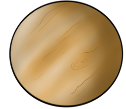
IŪPPITER
